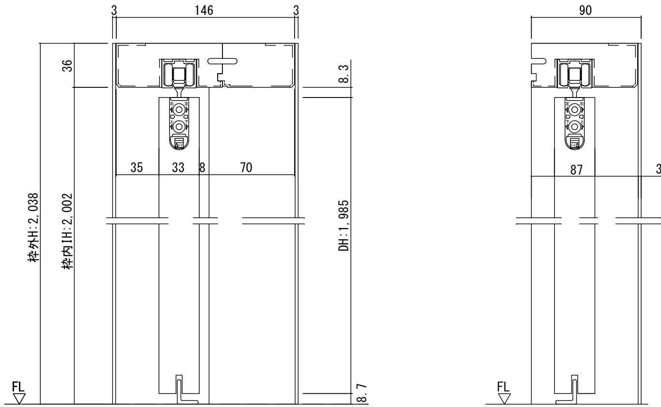
断面図
